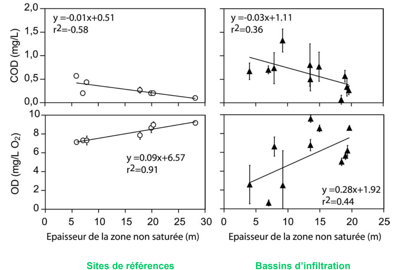
Figure 2. Relations entre les concentrations en carbone organique dissous (COD) et en oxygène dissous (OD) dans les eaux souterraines et l'épaisseur de la zone non saturée à l'aplomb des sites de référence (panneaux de gauche) et des bassins d'infiltration (panneaux de droite).
